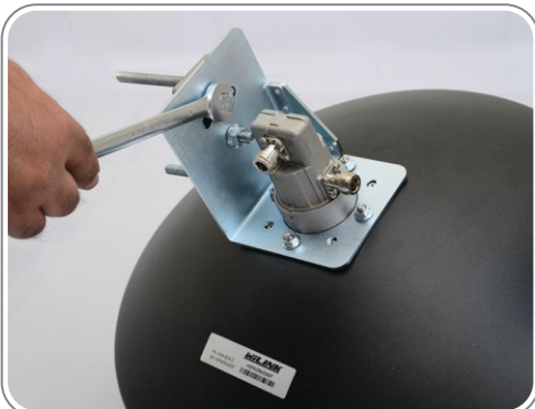
۸- نحوه بستن پیچ تنظیم به پایه و گیره لوله
