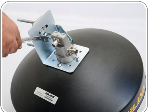
۷- نحوه بستن مهره اتصال دهنده پایه به گیره لوله
