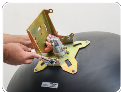
۳- نحوه اتصال براکت به پایه ستاره ای
