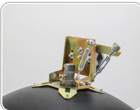
۱۴ - نمایی از آنتن مونتاژ شده بصورت کامل
