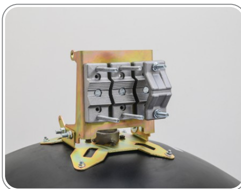
۸- بستن هر سه گیره
