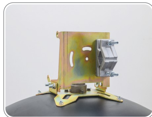
۷- نصب گیره لوله به پایه آنتن
