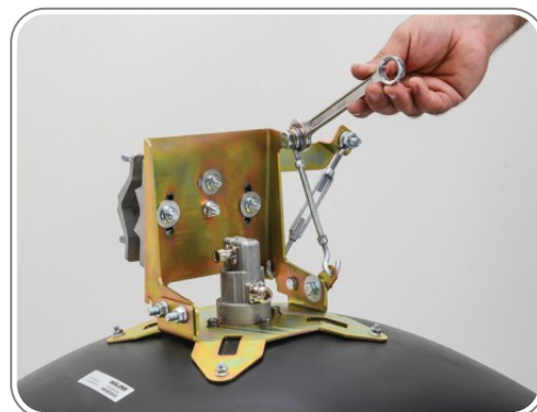
۱۳ - نصب مهارکش دوم جهت حرکت عمودی سر آنتن به صورت میلیمتری (Fine Tune)
