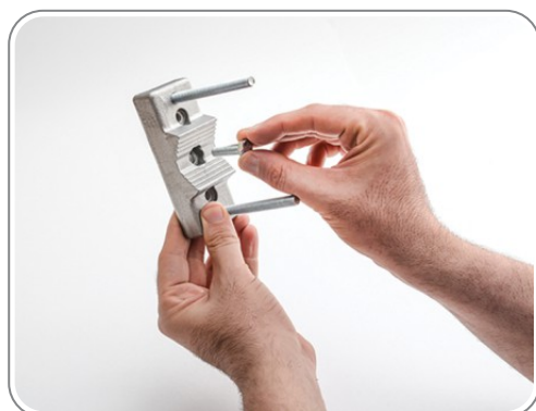
۶- نحوه قرار دادن پیچ مرکزی درون گیره لوله
