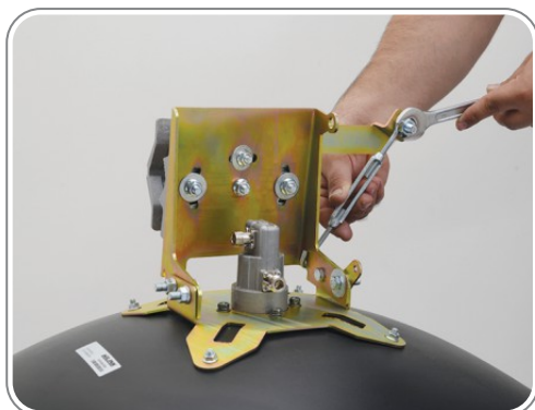
۱۲ - نصب مهارکش اول جهت حرکت عمودی سر آنتن به صورت میلیمتری (Fine Tune)
