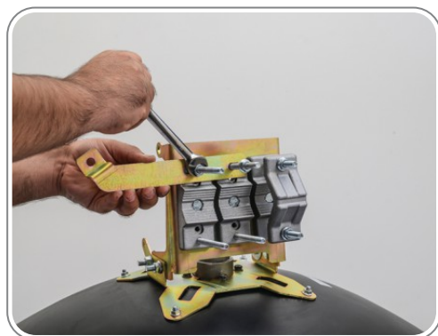
۹- نحوه نصب قطعه مخصوص اتصال مهارکش
