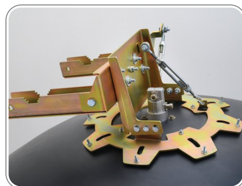
۱۰ - نمای کلی پس از نصب متعلقات آنتن
