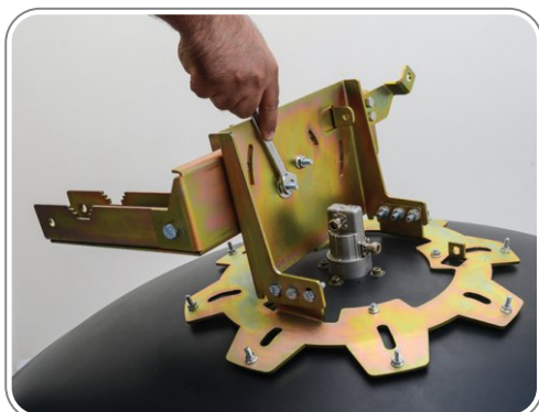
۳- نحوه قرار گرفتن پایه خرچنگی به براکت
