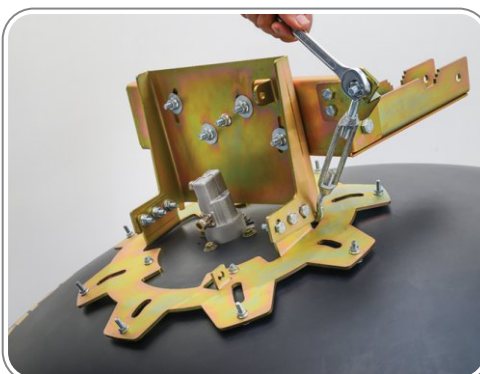
۷- نمای کلی از بستن پیچ های تنظیم
