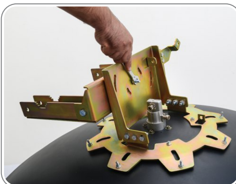
۴- نحوه بستن پایه خرچنگی به براکت با پیچ رابط
