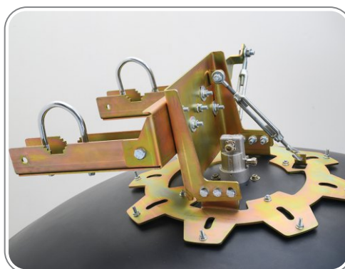
۱۱ - محل و نحوه نصب کُرپی‌ها، جهت اتصال آنتن به لوله دکل
