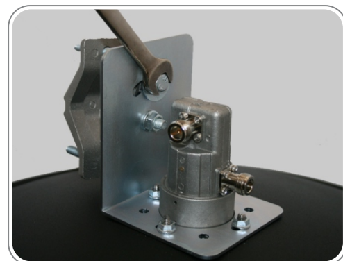
۱۰ - نحوه بستن پیچ تنظیم به گیره لوله
