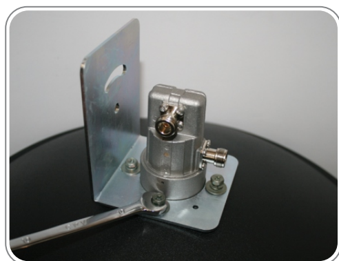
۶- نحوه بستن پایه و فیذ به دیش
