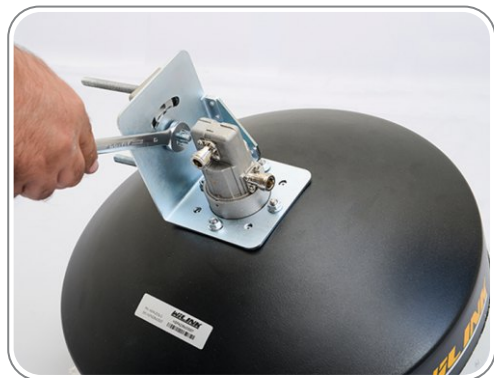
۹- نحوه بستن گیره لوله به پایه آنتن
