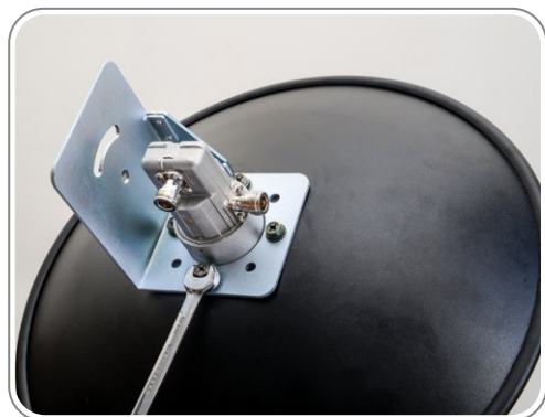
۶- نحوه بستن پایه و فید به دیش
