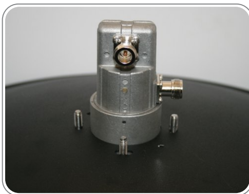
۵- نحوه قرار گرفتن فید بر روی آنتن از پشت
