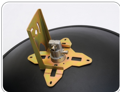
۶- نحوه قرار گرفتن پایه و فید روی دیش
