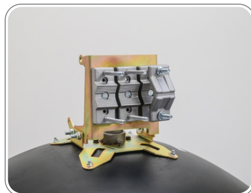
۱۰ - بستن هر سه گیره
