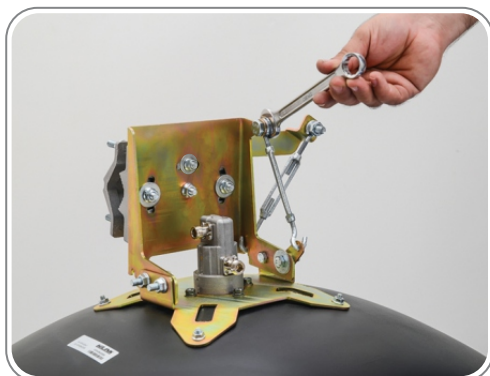
۱۵ - نصب مهارکش دوم جهت حرکت عمودی سر آنتن به صورت میلیمتری (Fine Tune)
