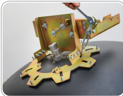
۸- نصب مهرکش اول جهت حرکت عمودی سر آنتن دیش به صورت میلیمتری (Fine Tune)
