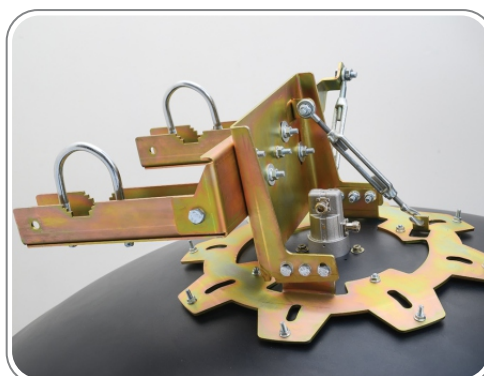
۱۲ - نحوه نصب کرپی ها جهت اتصال آنتن به دکل
