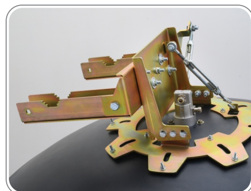
۱۰ - نحوه قرار گرفتن متعلقات آنتن
