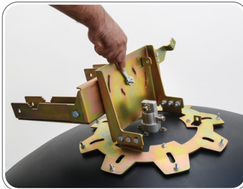
۵- محکم کردن مهره پیچ رابط پایه خرچنگی به پایه
