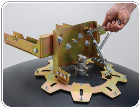
۷- نحوه محکم کردن همه پیچ و مهره های متحرک
