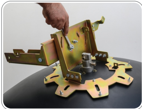
۴- محل نصب پیچ رابط پایه خرچنگی به پایه
